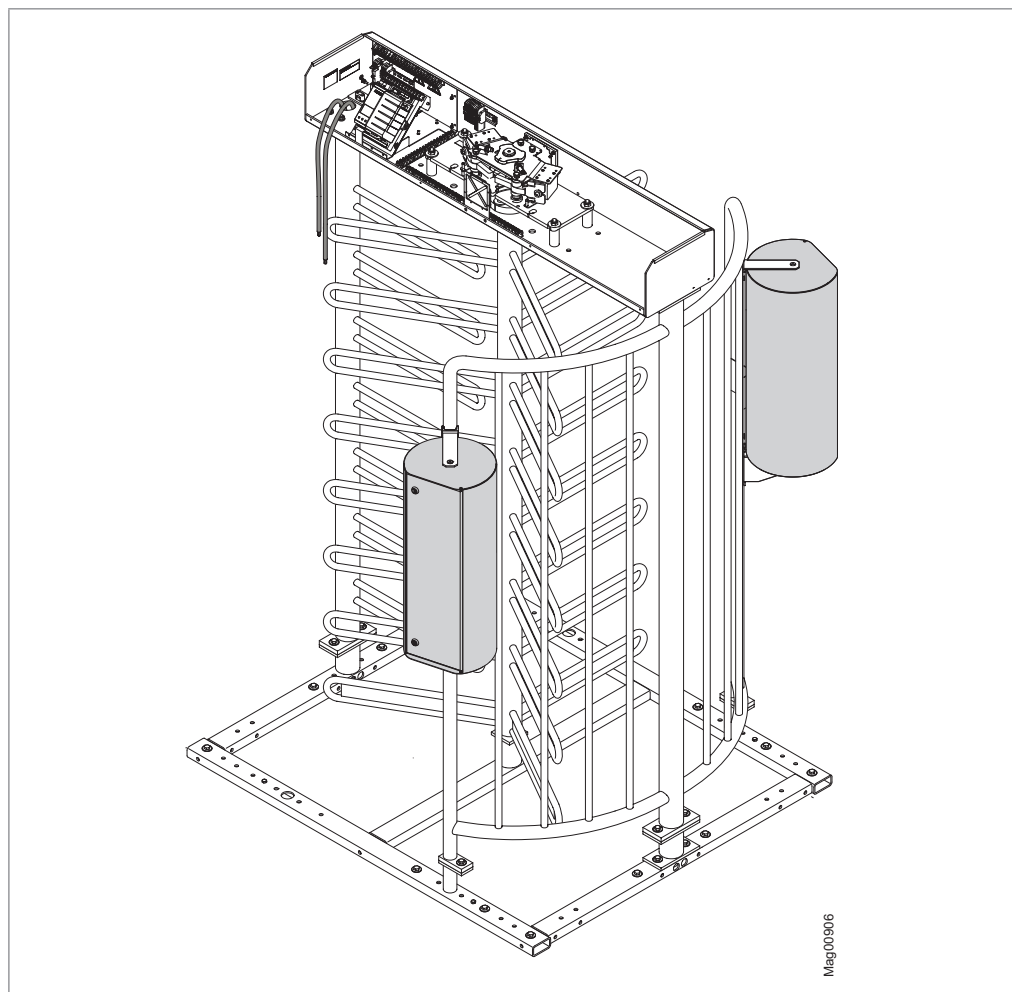
Fig. 43: Optional mounting pillars
